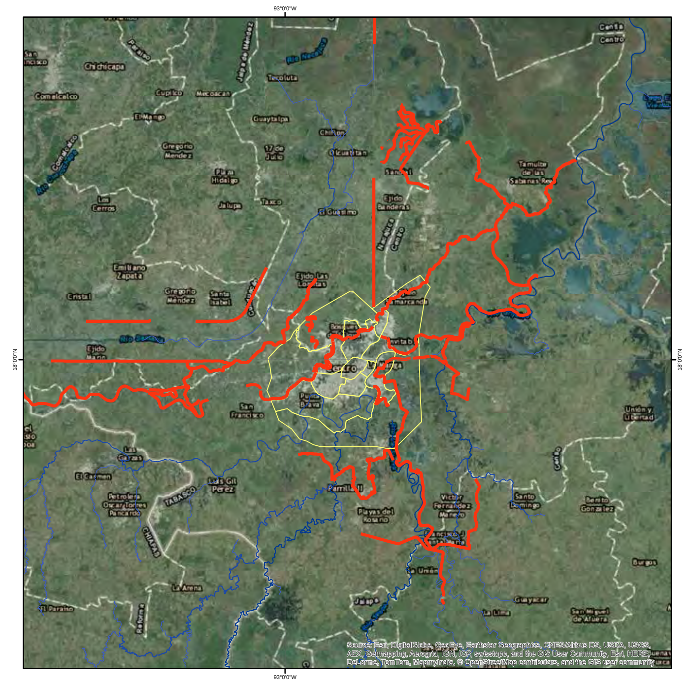
Figura 5.2.44. Distribución de las principales estructuras para el control de las inundaciones. El total de kilómetros de bordos y bardas de protección contabilizados para este trabajo rebasan los 378 km.
